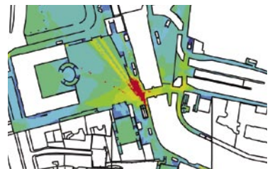
Isovistanalys - överblickbarhet vid Slussens torgplan (Spacescape AB 2007)
